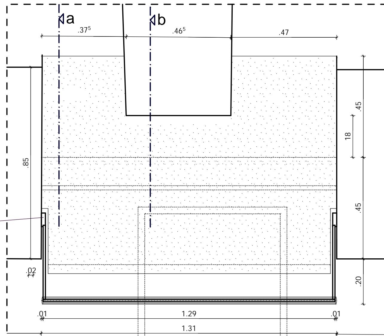
GR im Vitrinenbereich M 1 : 10
