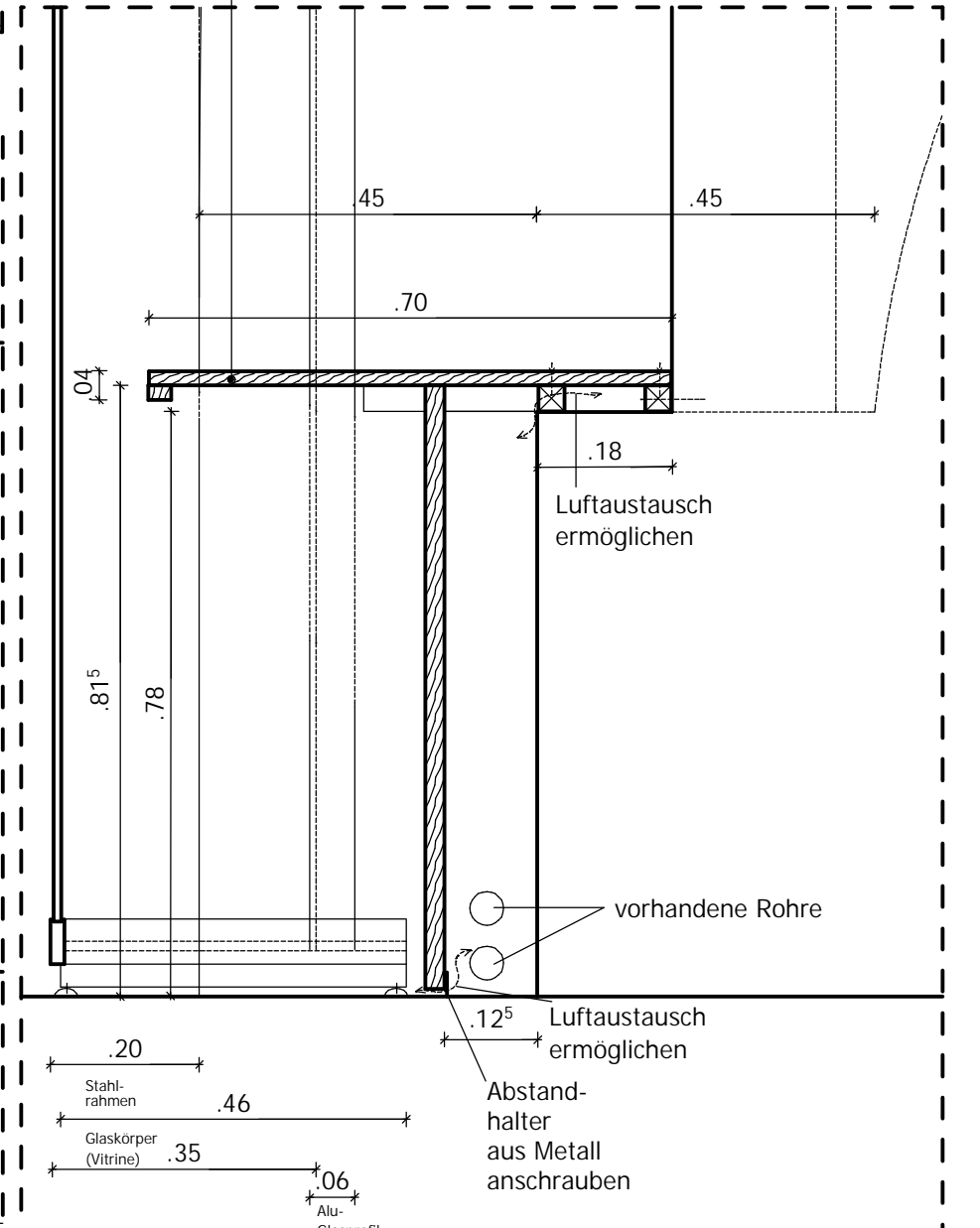
Schnitt b M 1 : 10
