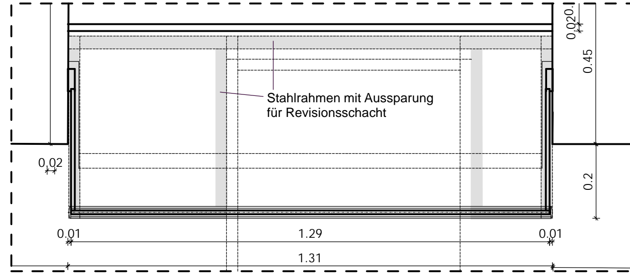
GR Fußpunkt Vitrine M 1 : 10
