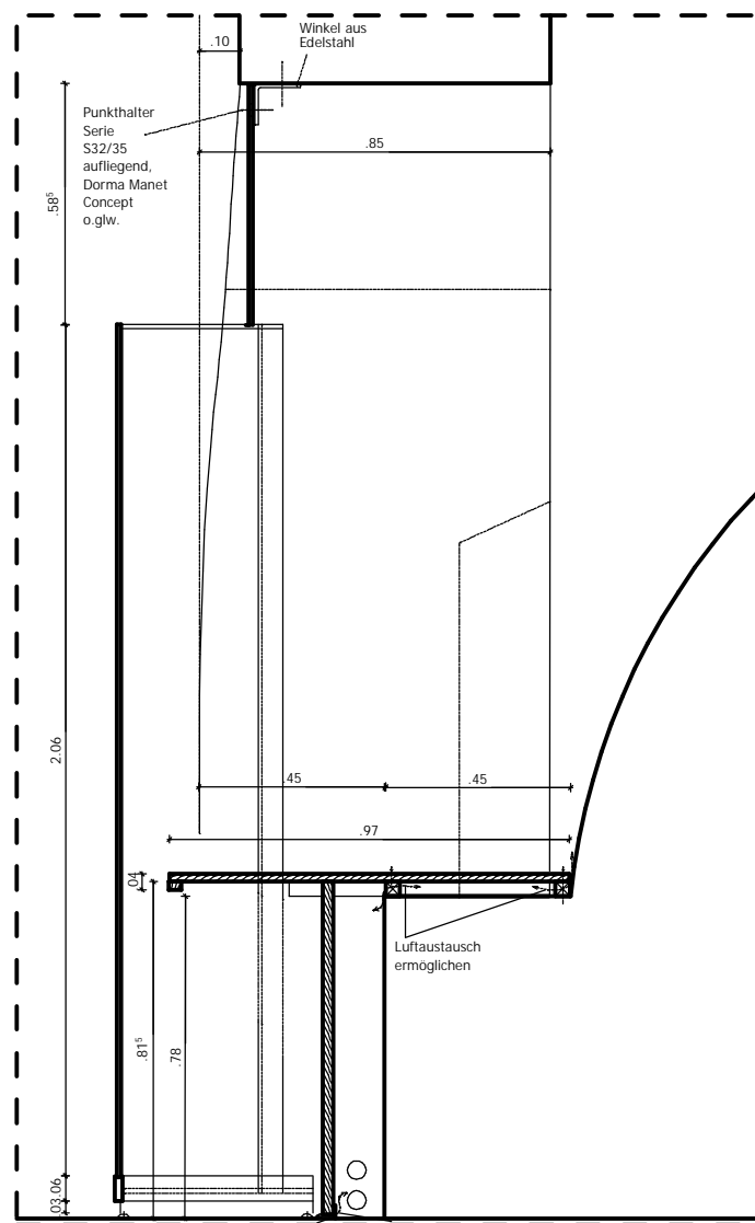
Schnitt a M 1 : 20
