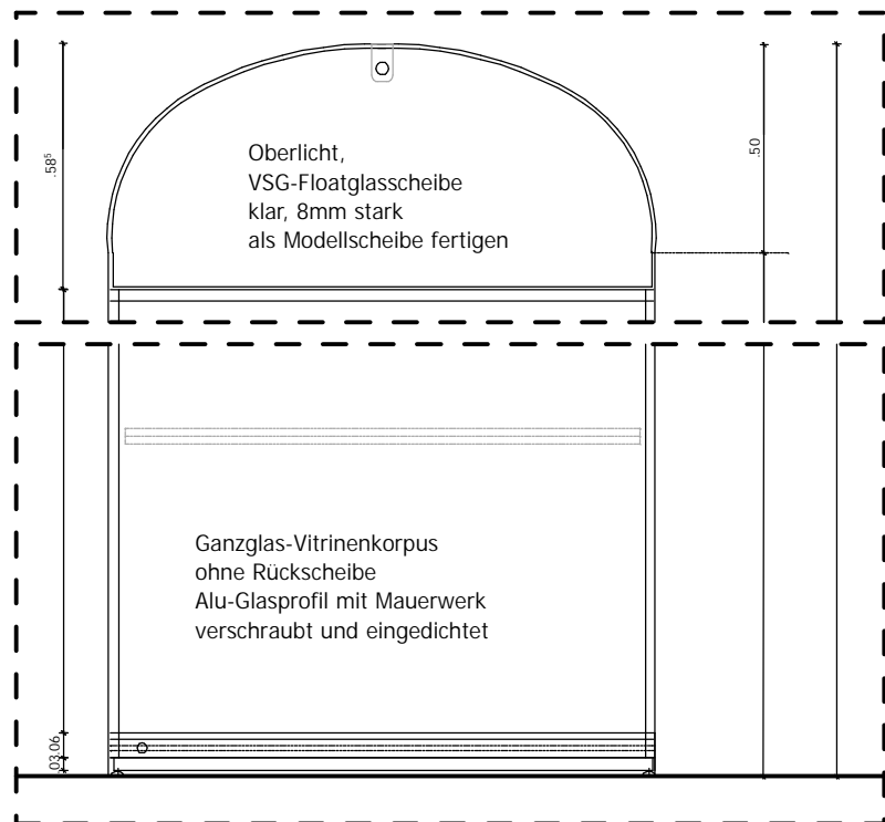
Ansicht M 1 : 20
